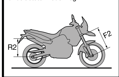
unbelasteter Federweg
